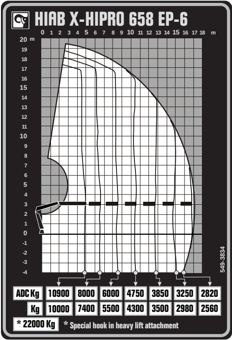
Diagrama de carga HIAB X-HIPRO 658 EP-6
