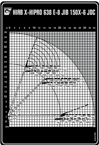
Diagrama de carga HIAB X-HIPRO 638 E-8 JIB150X-6
